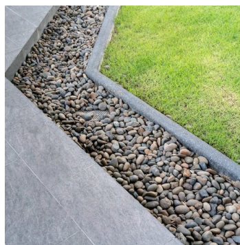
Рисунок 2. Дренажная полоса из гравия.
